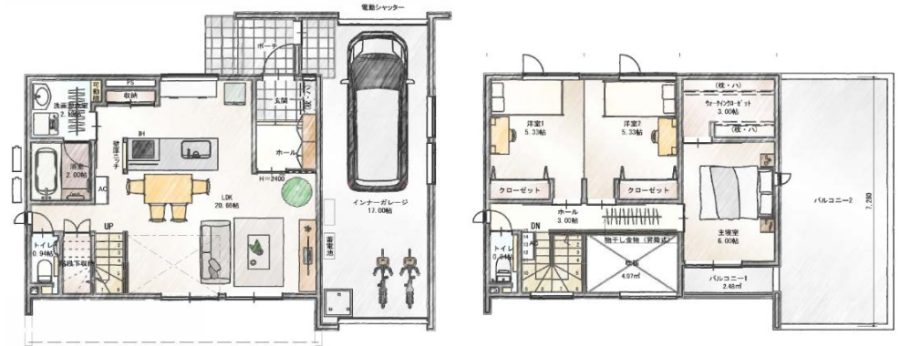
1階平面図
